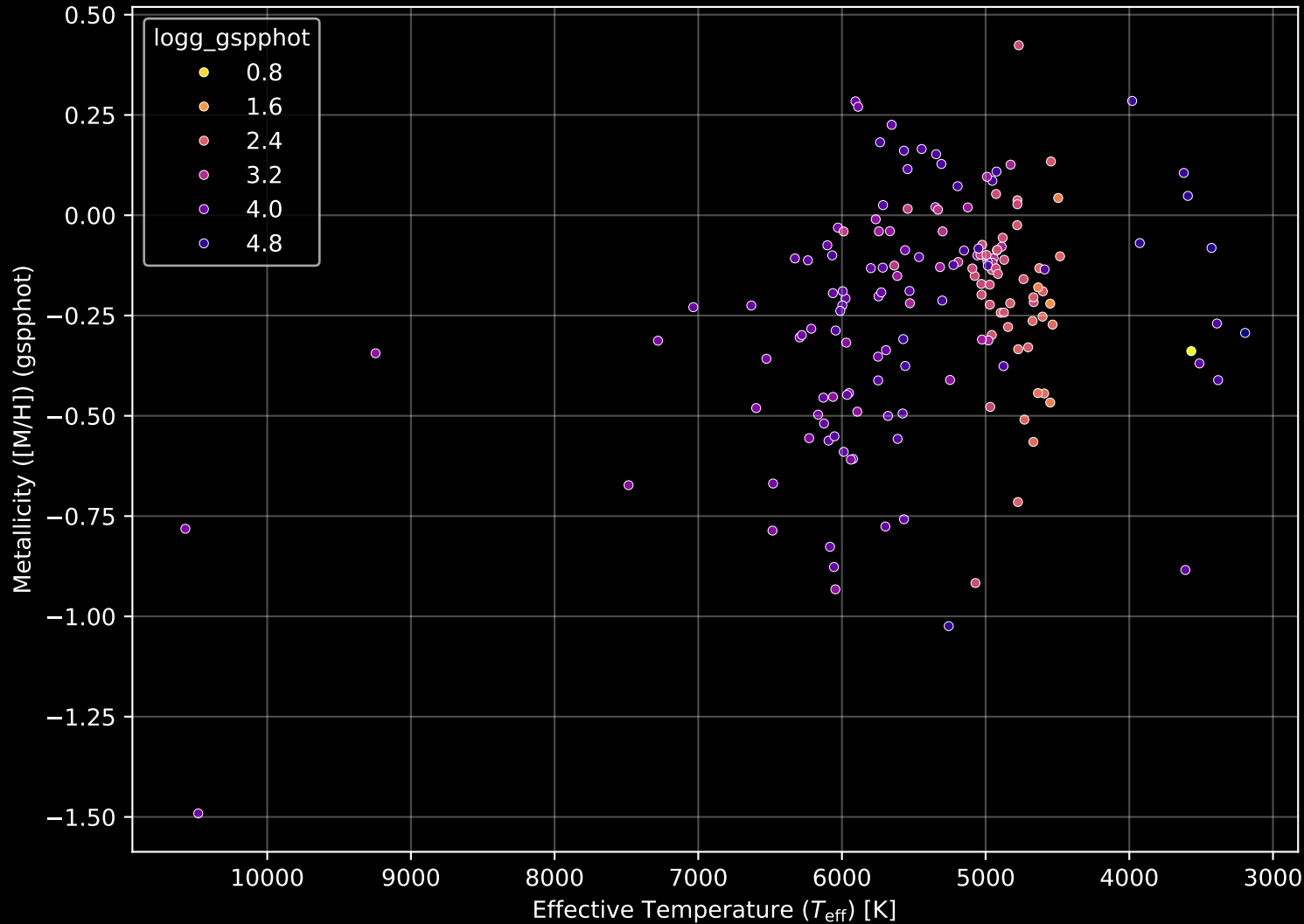
APOGEE DR17 Field: [266-24-O_TESS] Stellar Population Parameters (n= 166)
